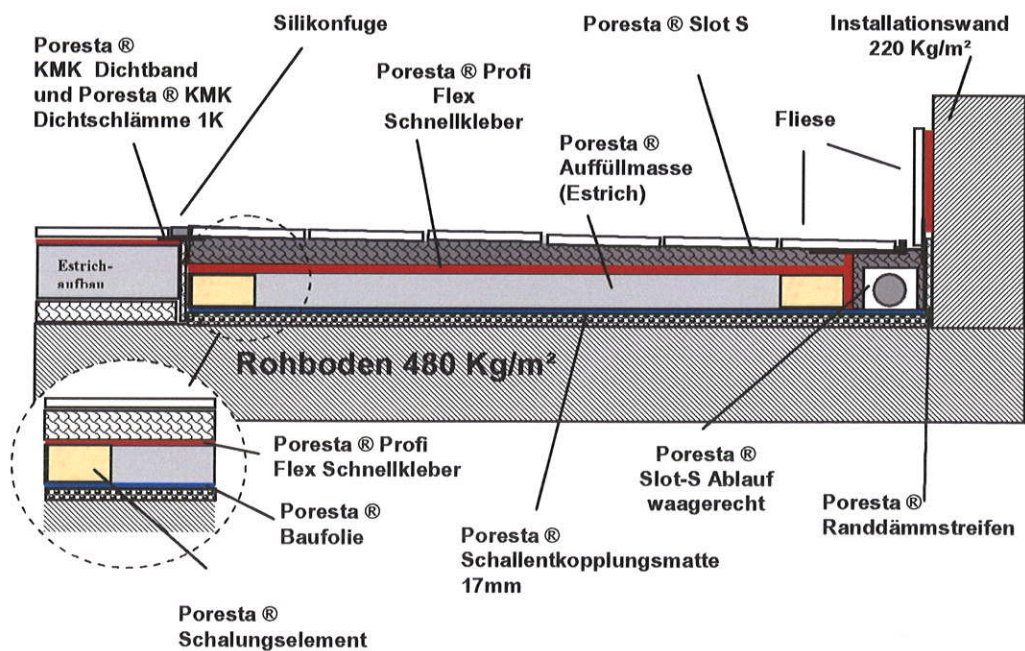
Bild 2 Auf dem Rohboden angebrachtes "Poresta® Schallschutzset BEDS Komplettset 2" für bodenebene Duschsysteme in Verbindung mit dem verfliesbaren Duschsystem "Poresta® Slot S" der Firma illbruck Sanitärtechnik GmbH, im Installationsraum (oben) und Schnittzeichnung mit Estrichanschluss (unten, Zeichnung des Auftraggebers).
